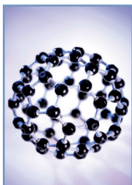
ii) Fulereno
