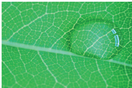
Efeito lótus
