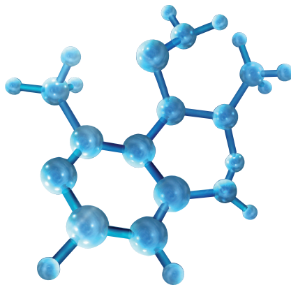
Nanotecnologia: mundo dos átomos e moléculas
