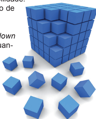
Blocos de construção e o sistema auto-organizado
